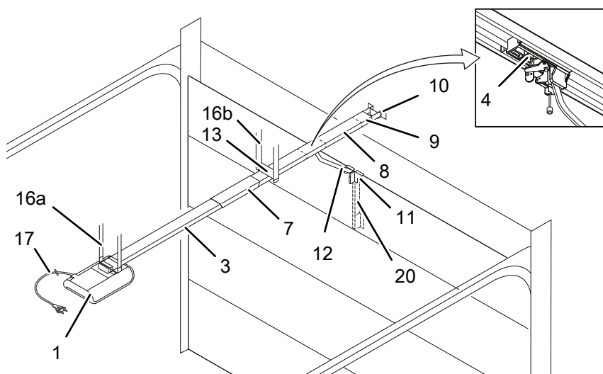
Obr. 1: Přehled produktu
