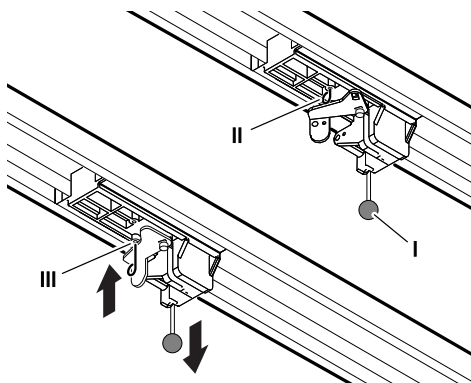
Rys. 6: Wysprężanie i zasprężanie napędu
