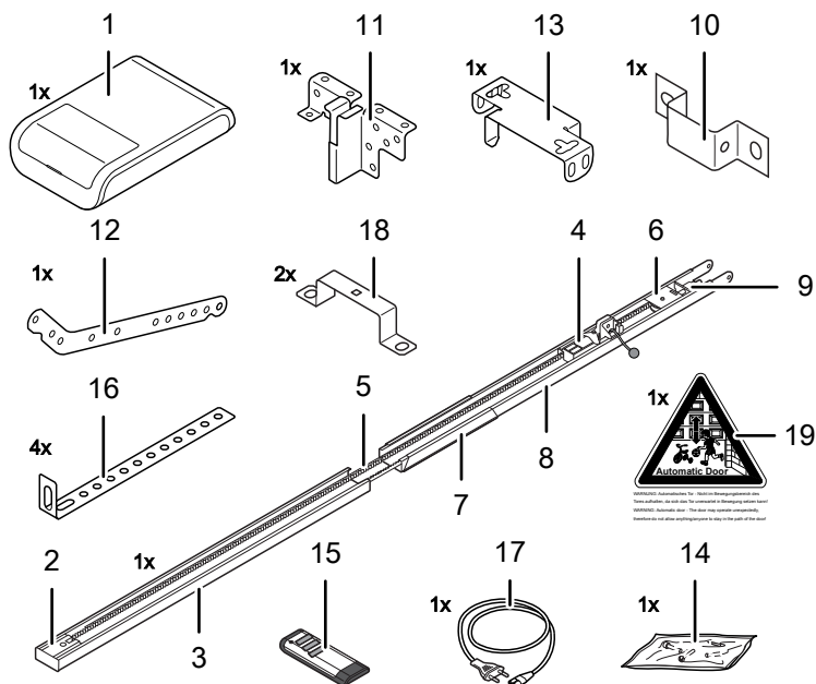
Obr. 4: Rozsah dodávky
