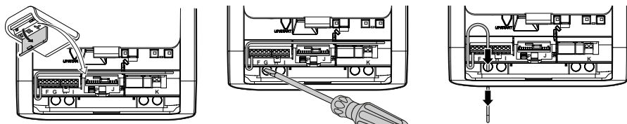
Kuva 8: Antennin asentaminen
