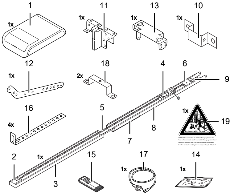
Kuva 4: Toimituksen sisältö
