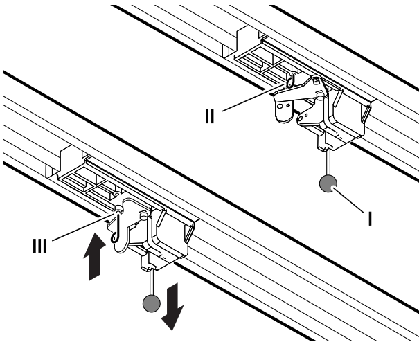
Fig. 16: Låsa upp och låsa drivenheten
