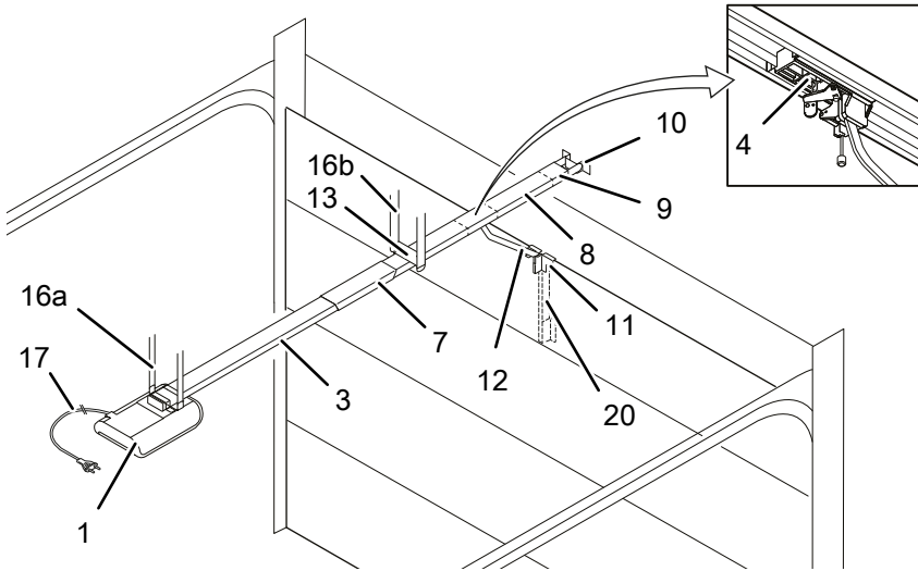
Fig. 1: Produktöversikt
