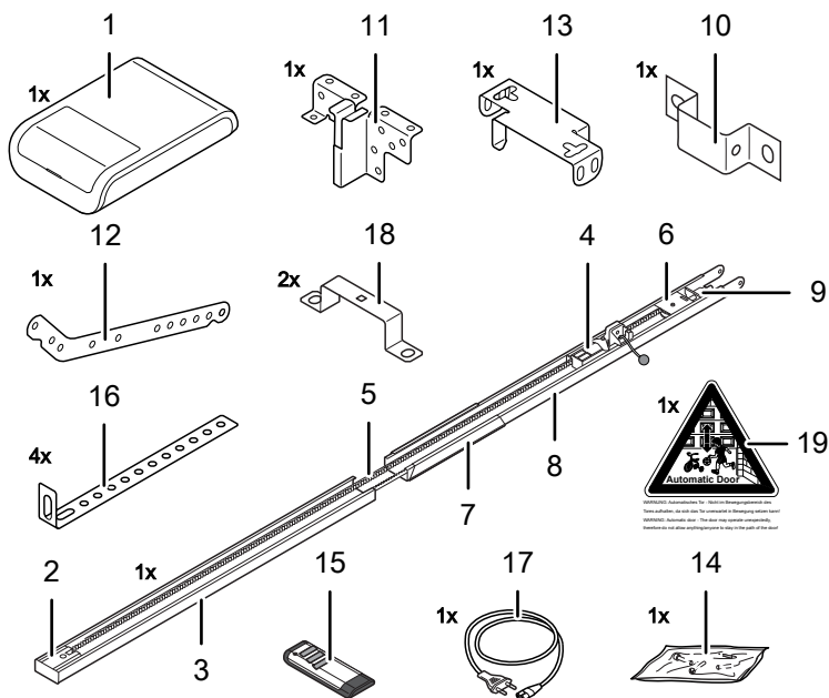
Fig. 4: Leveransomfattning
