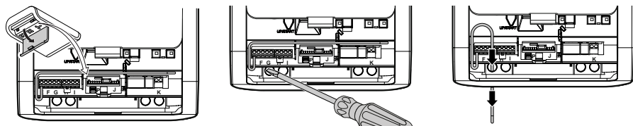
Obr. 8: Umístění antény
