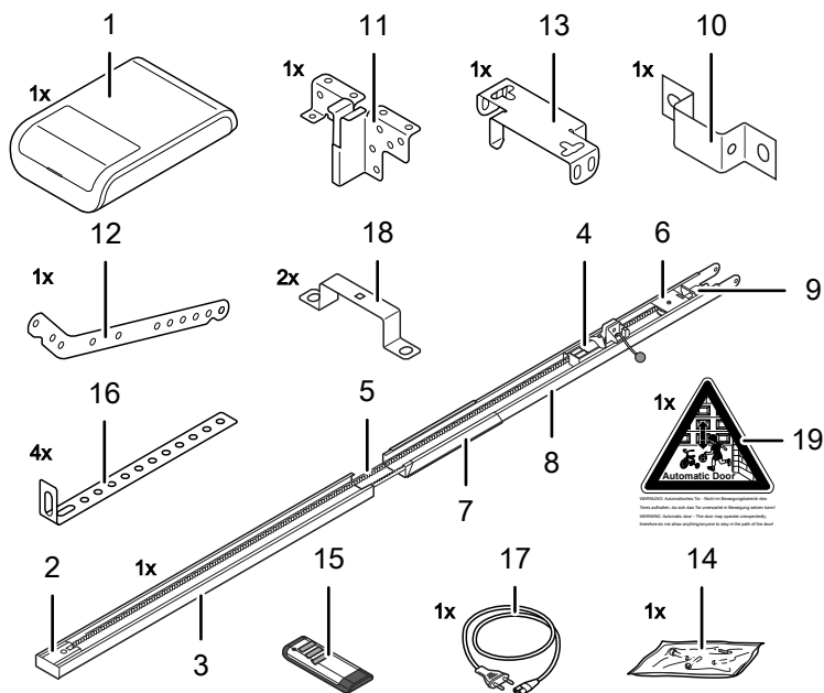
III. 4: Leveringsomfang
