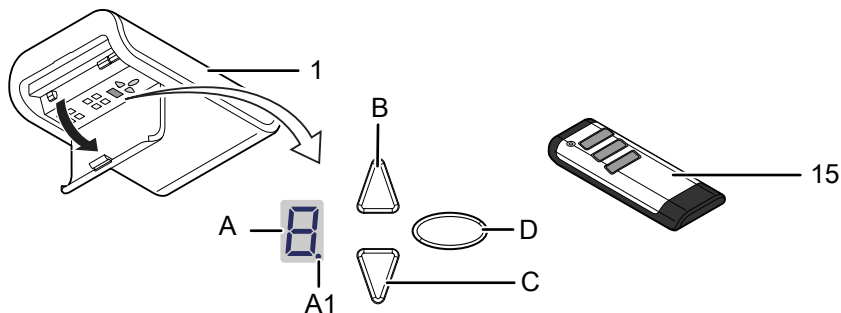
Obr. 2: Ovládací prvky
