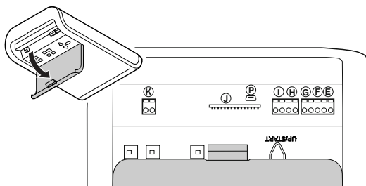
Obr. 7: Otevřete kryt hnací hlavy
