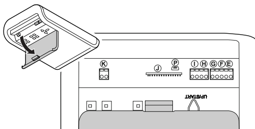
Fig. 7: Öppna drivhuvudets skydd
