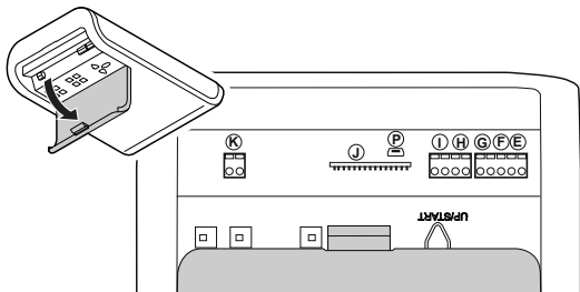
Rys. 7: Otwieranie pokrywy głowicy napędowej
