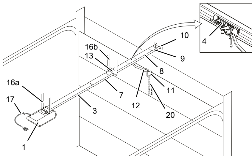
Rys. 1: Widok urządzenia
