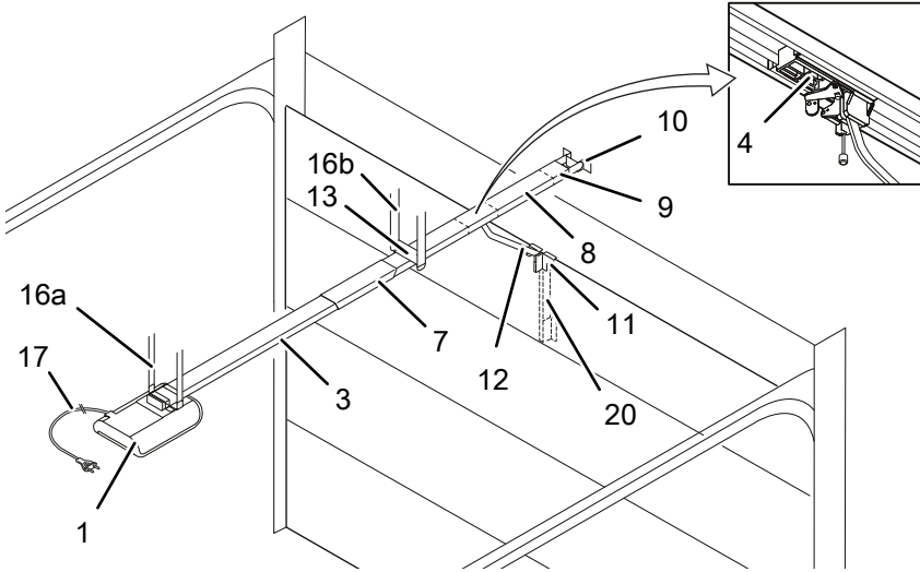
Kuva 1: Yleiskuva tuotteesta
